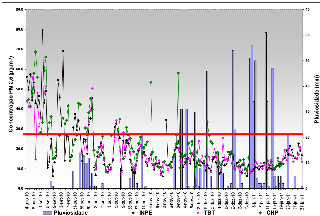
Figura 3 - Valores médios diários de material particulado fino, 2,5µm de diâmetro, e índice pluviométrico diário no período de 24 de agosto de 2010 a 25 de janeiro de 2011 nos municípios de São José do Campos, Cachoeira Paulista e Taubaté, Vale do Paraíba, SP. A linha vermelha na figura delimita o valor máximo diário recomendado pela OMS
